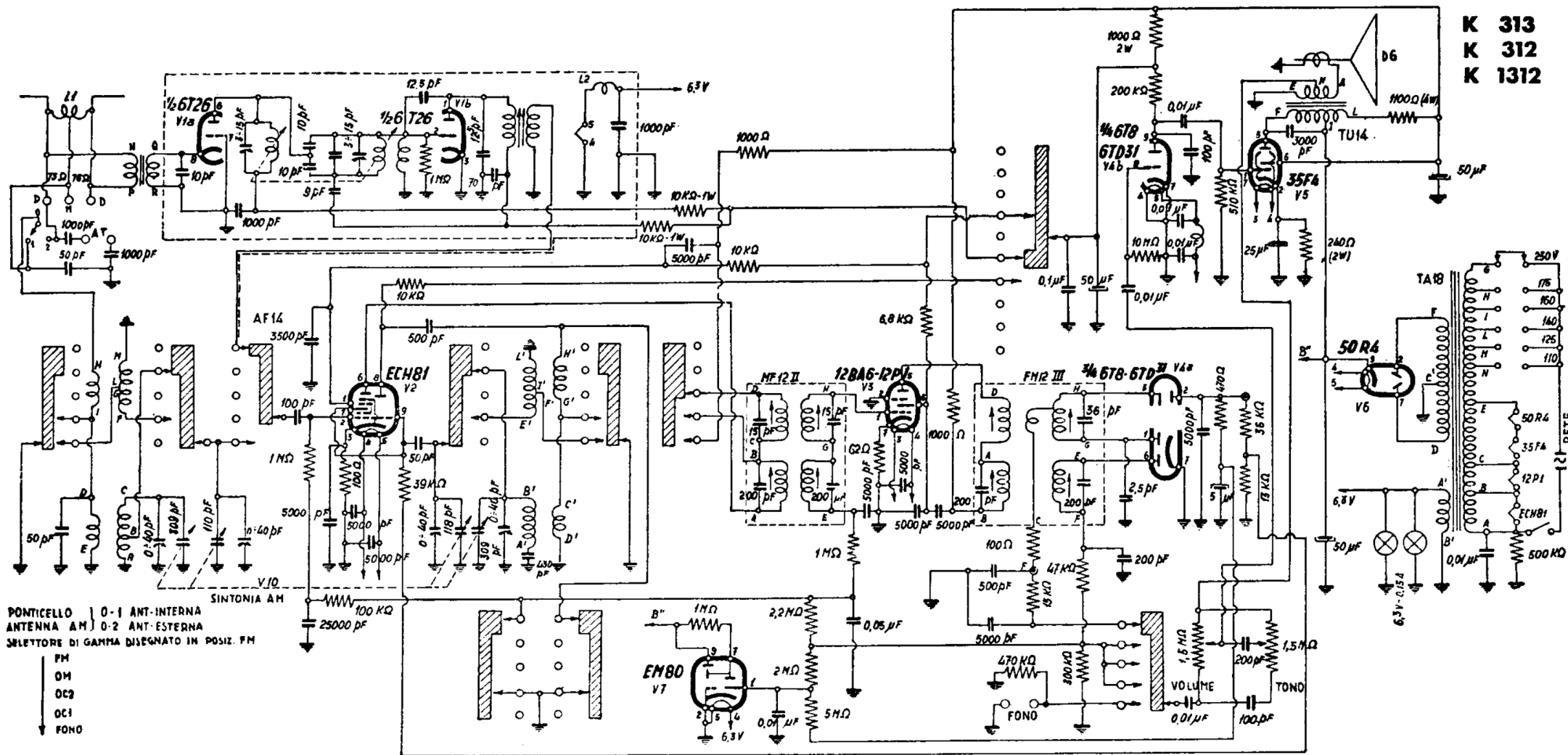
MAGNADYNE RADIO - Modd. FM 12, FM 13, FM 112 e FM 113, K 312, K 313, K 1312 e K 1313. Apparecchio a modulazione d'ampiezza e di frequenza, con gamma onde medie, due gamme onde corte e una banda onde ultracorte a modulazione di frequenza. Media frequenza AM a 471 kc/s, FM a 10,7 Mc/s. Potenza d'uscita 4 watt.
